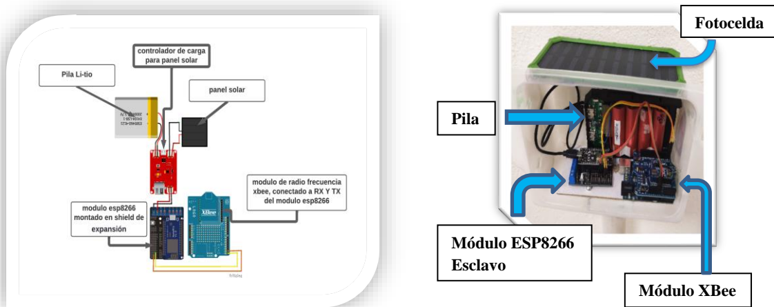
Figura 4. Diagrama esquemático y físico del módulo esclavo Fuente: Original
